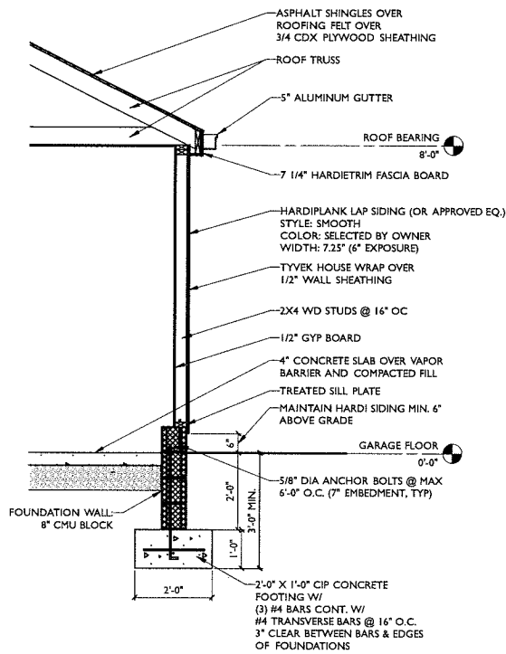
7 GARAGE SECTION Scale: 1/2" = 1'-0"
