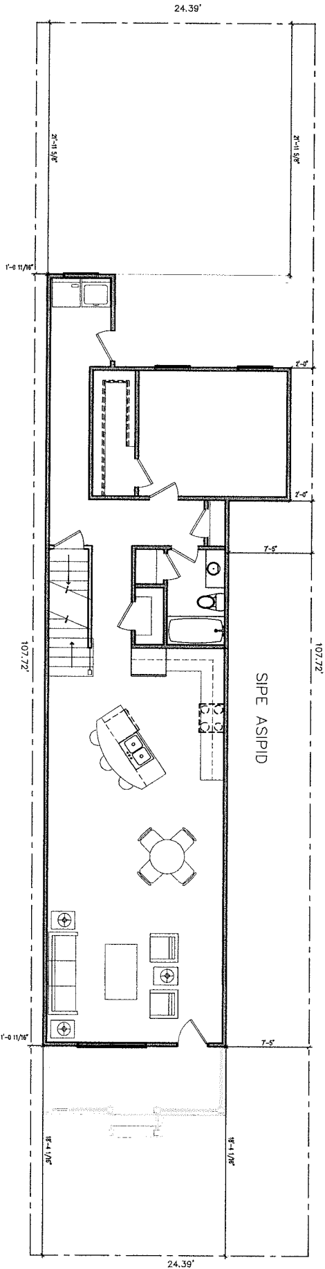
4 D-1 SCALE 1/4"=1'-0"
