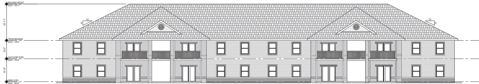
1 FRONT/REAR ELEVATION A1A SCALE: 1/8" = 1'-0"
