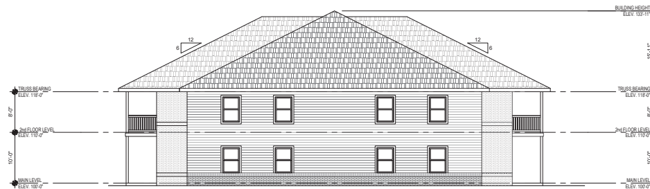
2 RIGHT/LEFT SIDE ELEVATION ATA SCALE: 1/8" = 1'-0"
