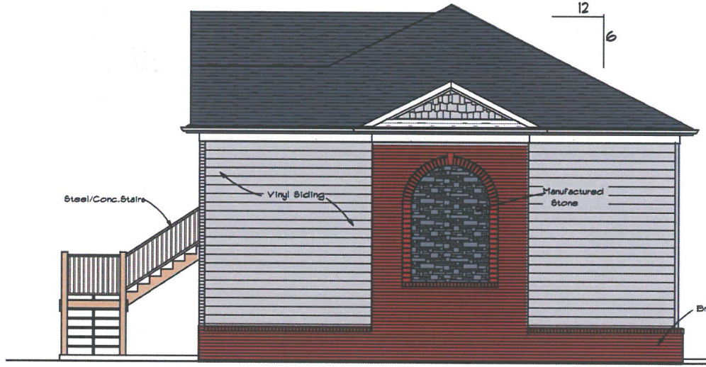
RIGHT ELEVATION
