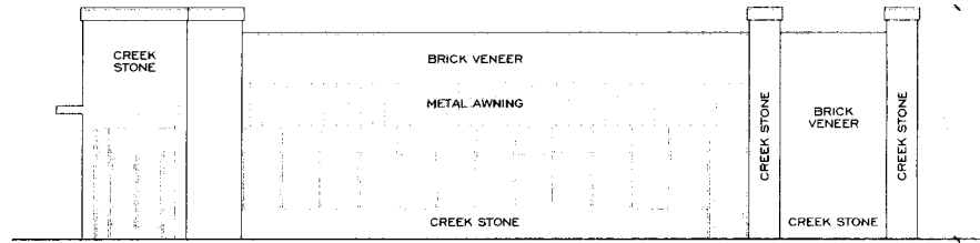
05 DIXIE ELEVATION A11 SCALE: 3/16" = 1'-0"
