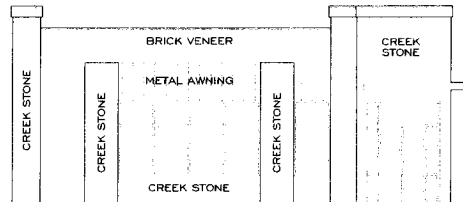
02 LUCAS ELEVATION A11 SCALE: 3/16" = 1'-0"
