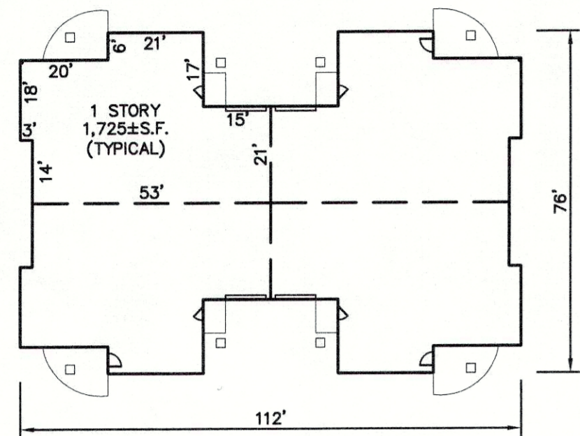
UNIT TYPE "A" SCALE: 1"=30'
