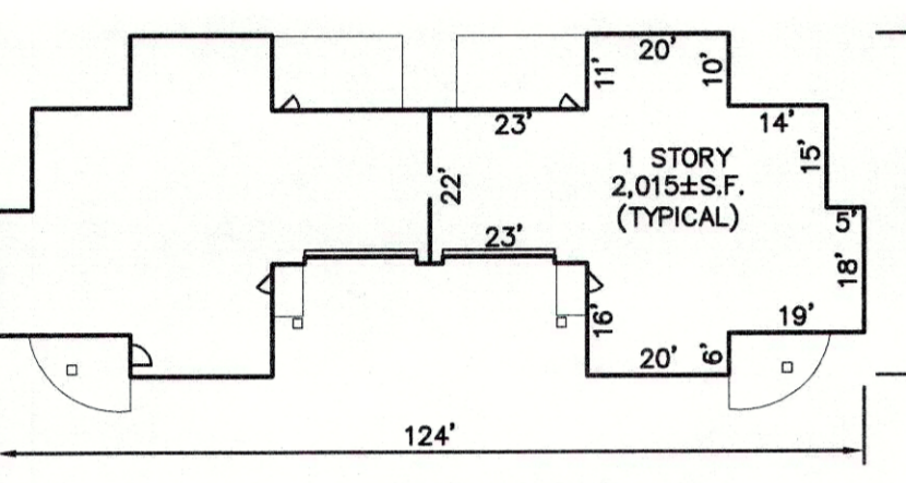
UNIT TYPE "B" SCALE: 1"=30'
