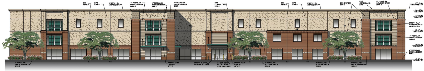
1 WEST ELEVATION SCALE: 1/8"=1'-0"
