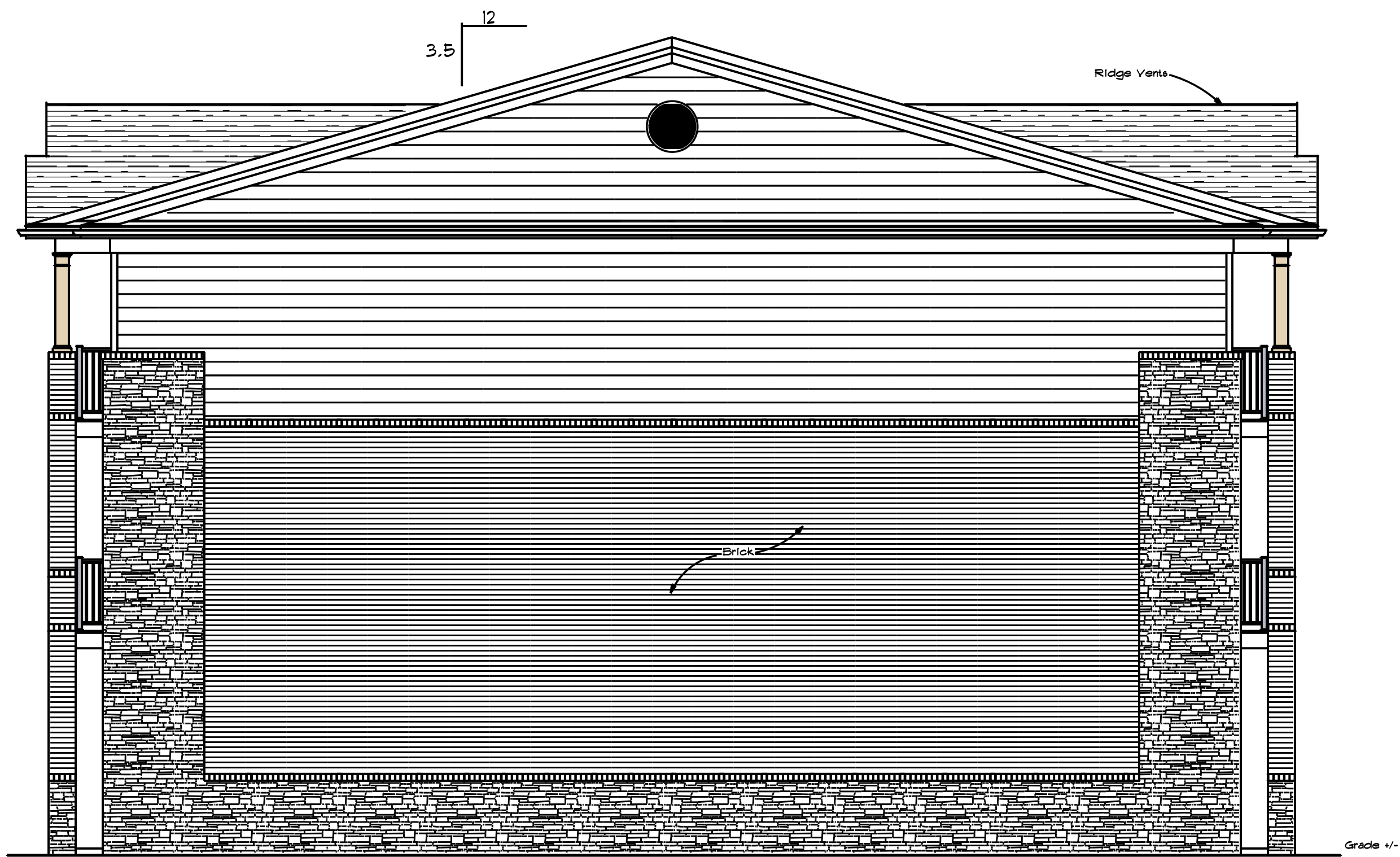
RIGHT ELEVATION
